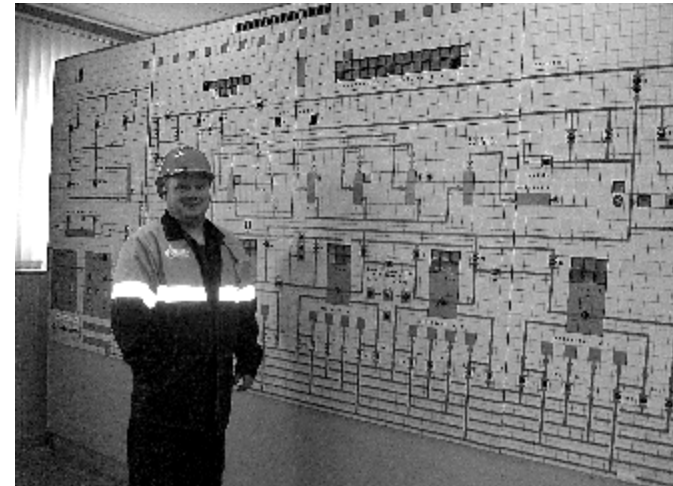
Помещение главного щита управления, откуда осуществляется контроль за работой всех агрегатов. За пультом - сменный инженер Сергей Петрович Назарук.
